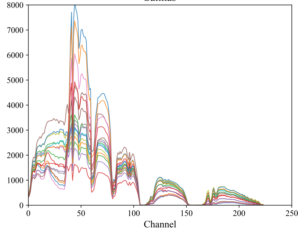
Salinas
